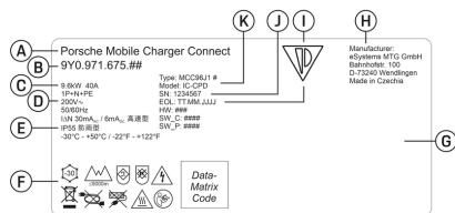
図. 13: 銘板 (例)
