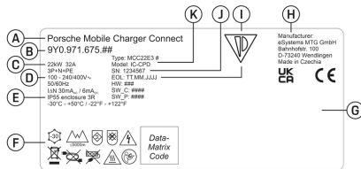
Abb. 12: Typenschild (Beispiel)
